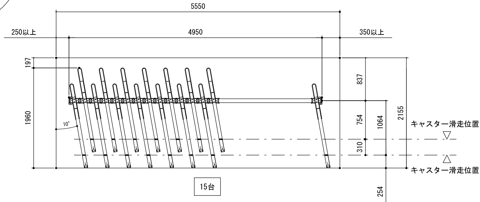
下段平面配置図 S=1/50
